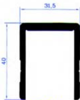
PA-211 Προφίλ Πι παραπέτων Βάρος: 880 gr/m
