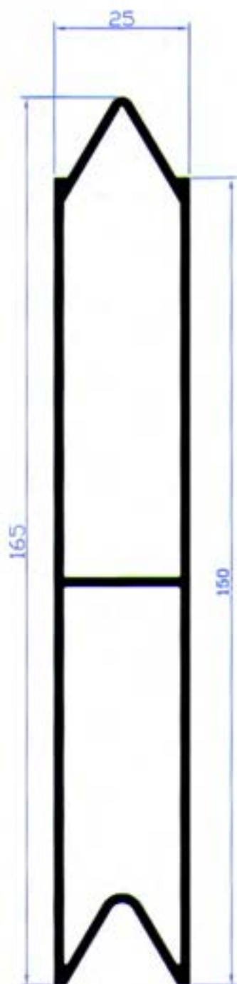
PA-223 Αντιανέμιο τέντας ραμποτέ Βάρος: 1742 gr/m
