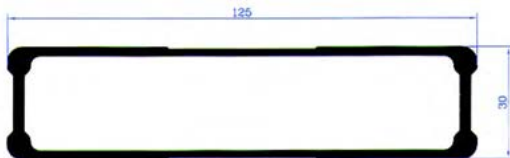
PA-221 Εξωτερικό προφίλ πτυσσόμενου συγκρατητή Βάρος: 2003 gr/m
