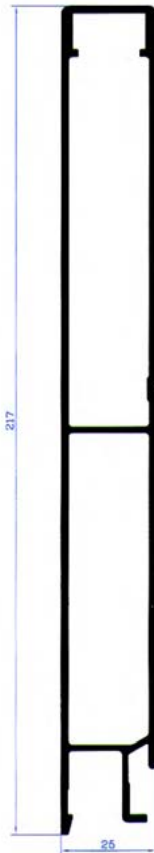
PA-201 Προφιλ κεφαλάρι Βάρος 2670 gr/m
