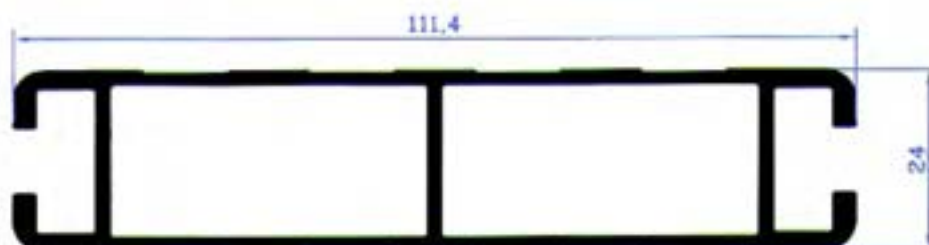
PA-222 Εσωτερικό προφίλ πτυσσόμενου συγκρατητή Βάρος: 1570 gr/m
