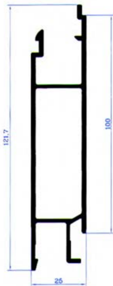
PA-205 Προφίλ μικρής σκάφης Βάρος: 2506 gr/m
